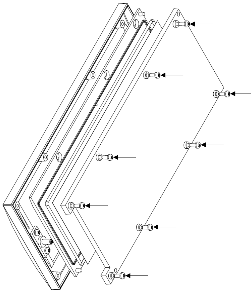
Ilustracja 1: Mocowanie docisku szybki
